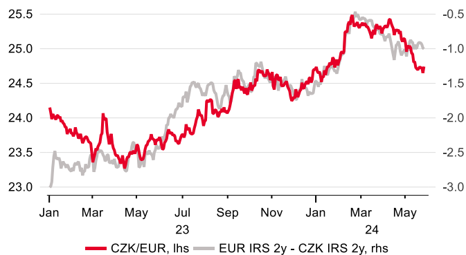
CZK/EUR a úrokový diferenciál
