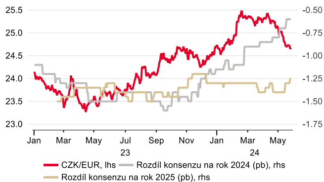
CZK/EUR a diferenciál růstu HDP mezi eurozónou a ČR
