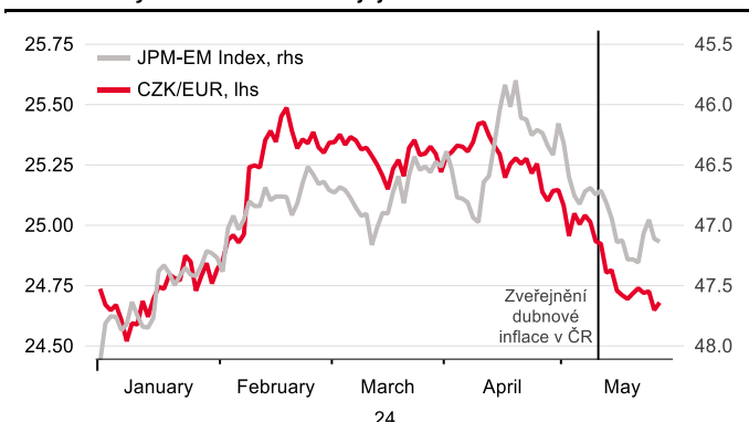
Kurz koruny a index měn rozvíjejících se trhů
